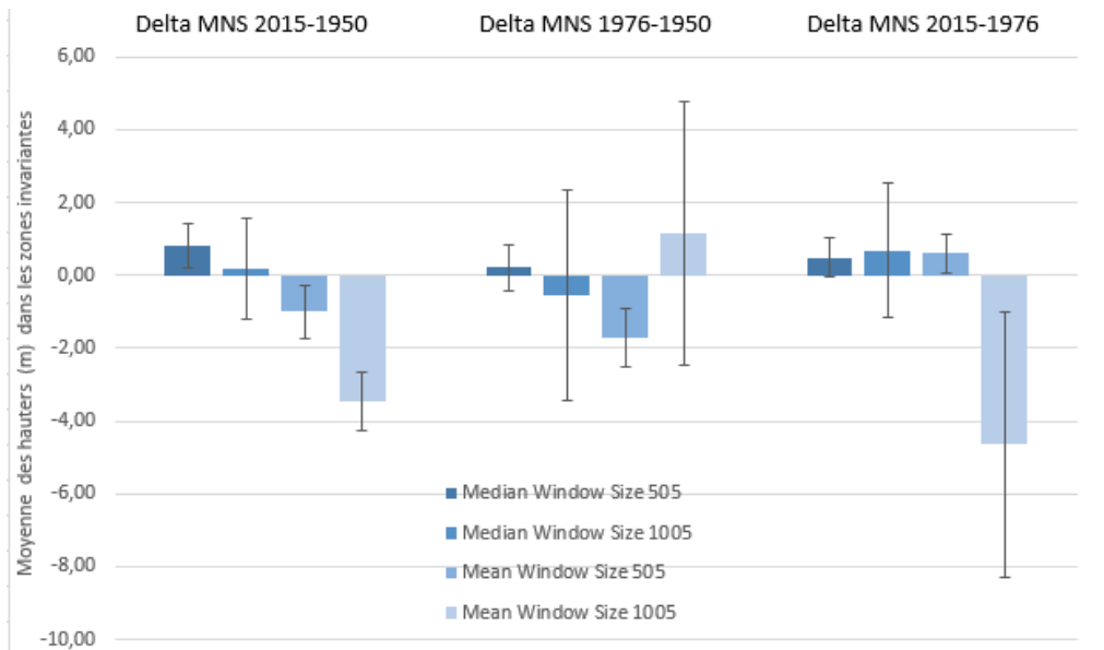
Fig. 38. Correction par statistiques focale dans les zones invariantes entre les trois dates.
