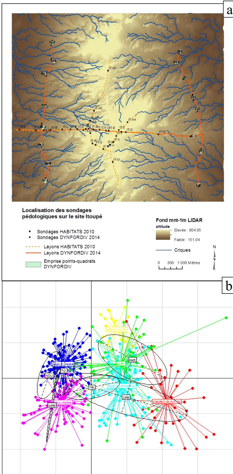
Fig 35. a) Localisation des relevés et des sondages pédologiques au site Itoupé (ITO). ; b) Situation pédologique des sites étudiés (ellipses) au regard de la diversité des sols forestiers de Guyane : projection des sondages sur l'espace multifactoriel (points de couleur et centroides par type de sol) d'une ACP tirée de Guitet et al. 2016.
