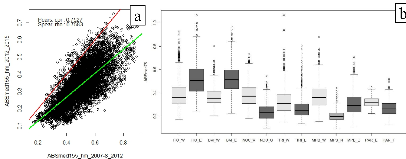
Fig. S4. a) Constance temporelle de la dynamique soulignée par la corrélation spatiale (trait vert) entre indicateurs pour deux périodes successives (2007-8 à 2012 et 2012 à 2015, site NOU) ; l'écart
