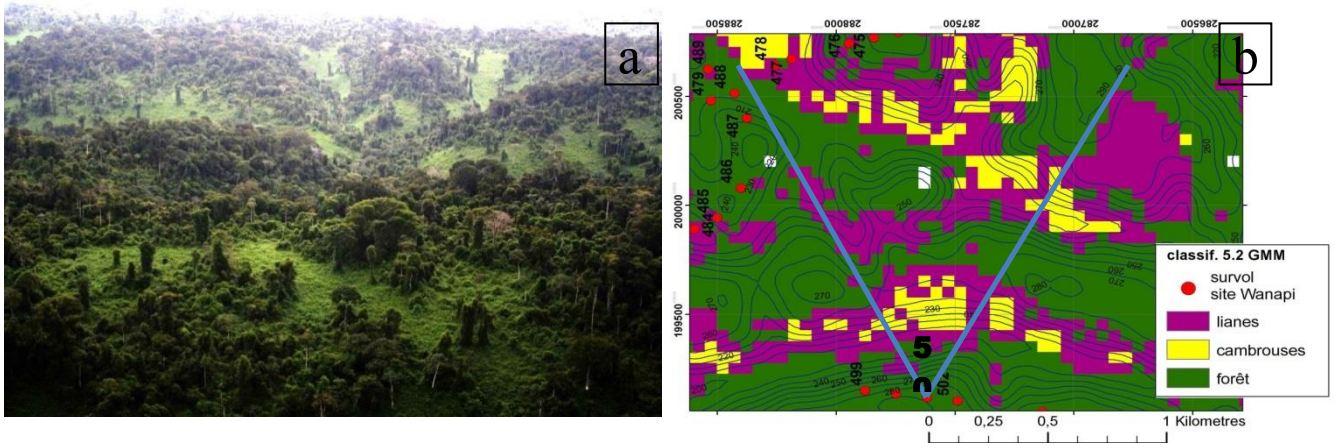
Fig. S7. a) Paysage à canopée ouverte, cambrouses et lianes au site Wanapi (photo n° 501 D. Sabatier) ; b) Extrait de la classification supervisée thématique de l’image Landsat au même site ; les lignes indiquent approximativement le champ de visée du cliché 501.
