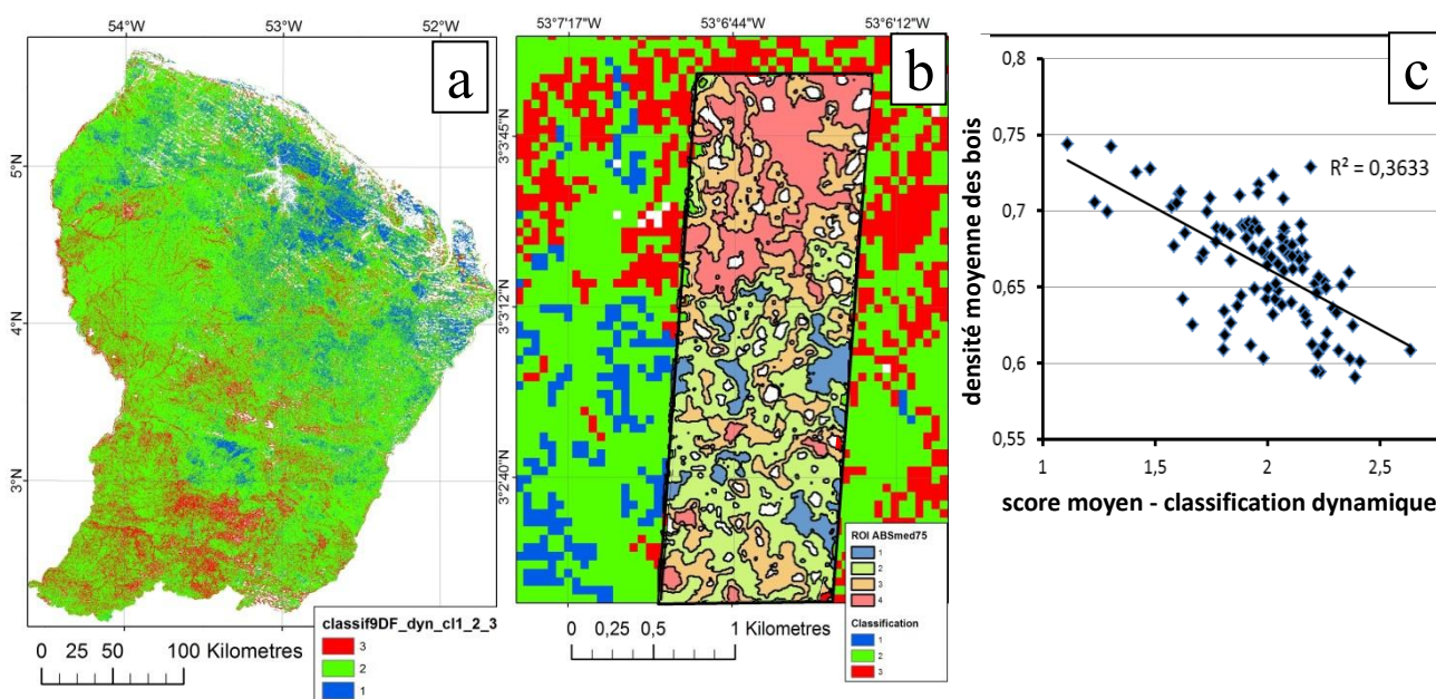
Fig. 10. a) Classification supervisée « dynamique » de l'image composite Landsat : trois classes de dynamique ; b) Zones d'apprentissage (ROI-dynamique) en 4 classes issues de l'analyse des données LiDAR (voir Fig. 3b) et classification après fusion des classes ROI 3 et 4 ; ITO-nord-ouest ; c) Relation densité des bois ~ dynamique par croisement des données Habitats et des scores de la classification supervisée dans un voisinage de 505 m.
