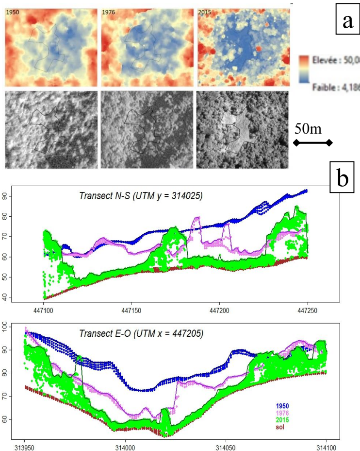
Fig. S10. a) Comparaison des modèles de canopée LiDAR (2015) et photogrammétriques (1950, 1976) mettant en évidence l'apparition d'une cambrouse ; haut : MNC 1950/1976/2015 ; bas : ortho-photos 1950/1976 et Pléiades 2014 ; b) Coupes nord-sud et est-ouest des modèles de canopée 1950, 1976 et 2015 ; les végétations basses correspondent à des cambrouses à bambous.
