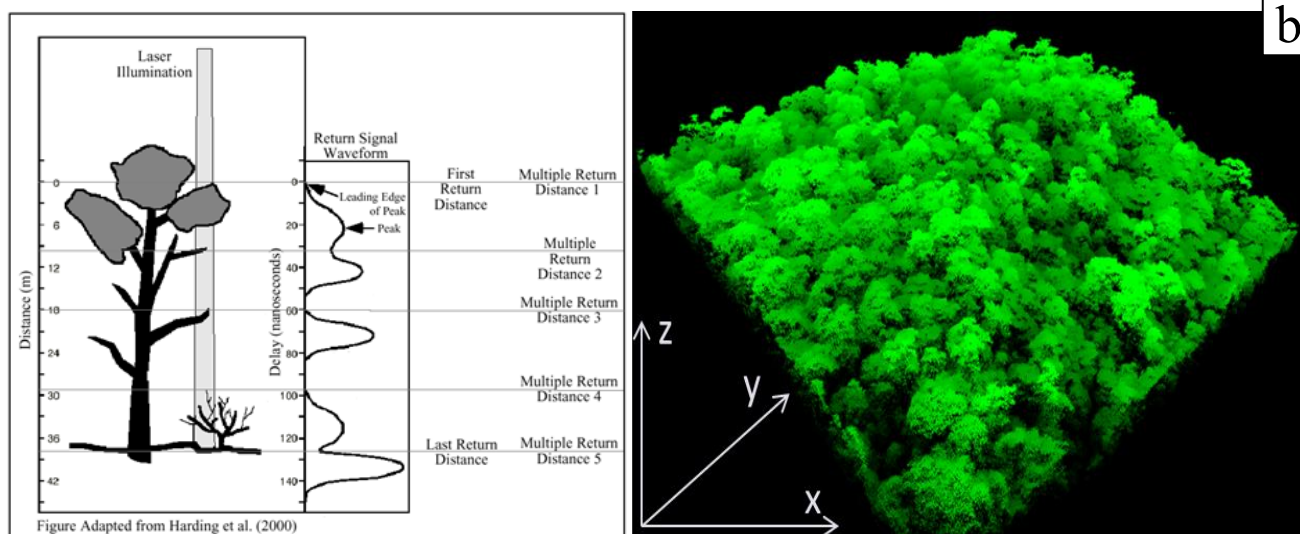
Fig. 31. Illustration de la technologie LiDAR ; a) Schéma du train d'onde généré par une impulsion, (adapté de Harding et al. 2000) ; b) Visualisation des données tridimensionnelles acquises sur la forêt.
