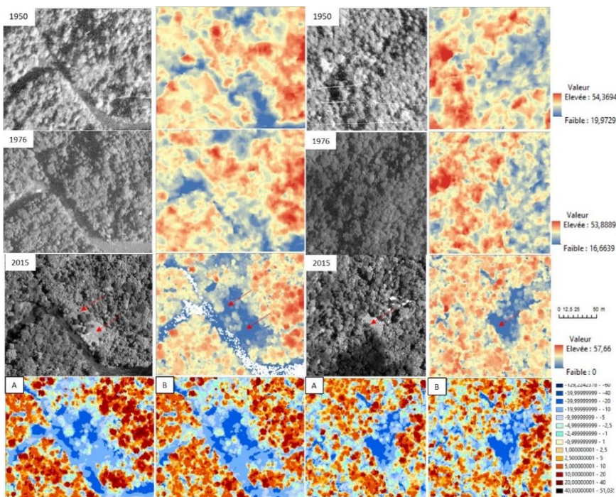
Fig. 40. Zones d'abatage des 2 camps et zones de posé d'hélicoptère. 1 ère /3 ème colonnes : extraits Ortho-photo 1950/1976 et Pléiades 2014. 2 ème /4 ème colonnes: extraits des MNC 1950/1976/2015 ; 4 ème ligne : delta des MNS A (2015-1950) ; B (2015-1976.). Echelle 1500.
