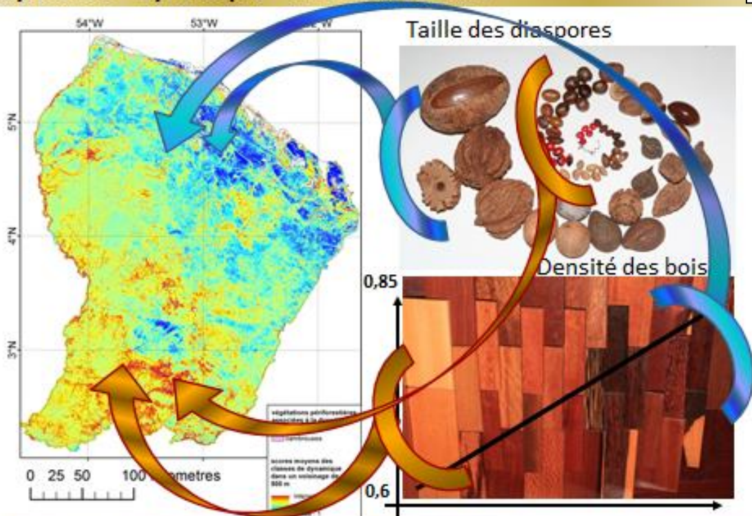
Fig. 23. a) Distribution des classes inférées de la classification « dynamique » de l'image Landsat dans les classes de paysages forestiers 18 à 22 (Gond et al. 2011) ; b) Représentation schématique de la biogéographie des arbres et des traits fonctionnels des communautés d'arbres en relation avec la dynamique forestière, utilisée à des fins didactiques.
