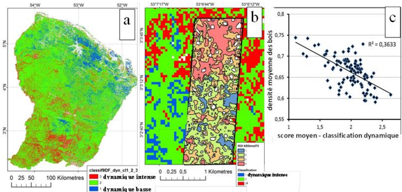
Fig. S8. a) Classification supervisée de l’image Landsat en trois classes de dynamique ; b) Zones d’apprentissage (ROI-dynamique) en 4 classes de l’indicateur ABSmed75 (voir Fig. 3b) superposées à la classification Landsat finale après fusion des classes 3 et 4 ; site ITO-nord-ouest ; c) Relation densité des bois ~ dynamique par croisement des données Habitats et des scores de la classification « dynamique » de l’image Landsat.
