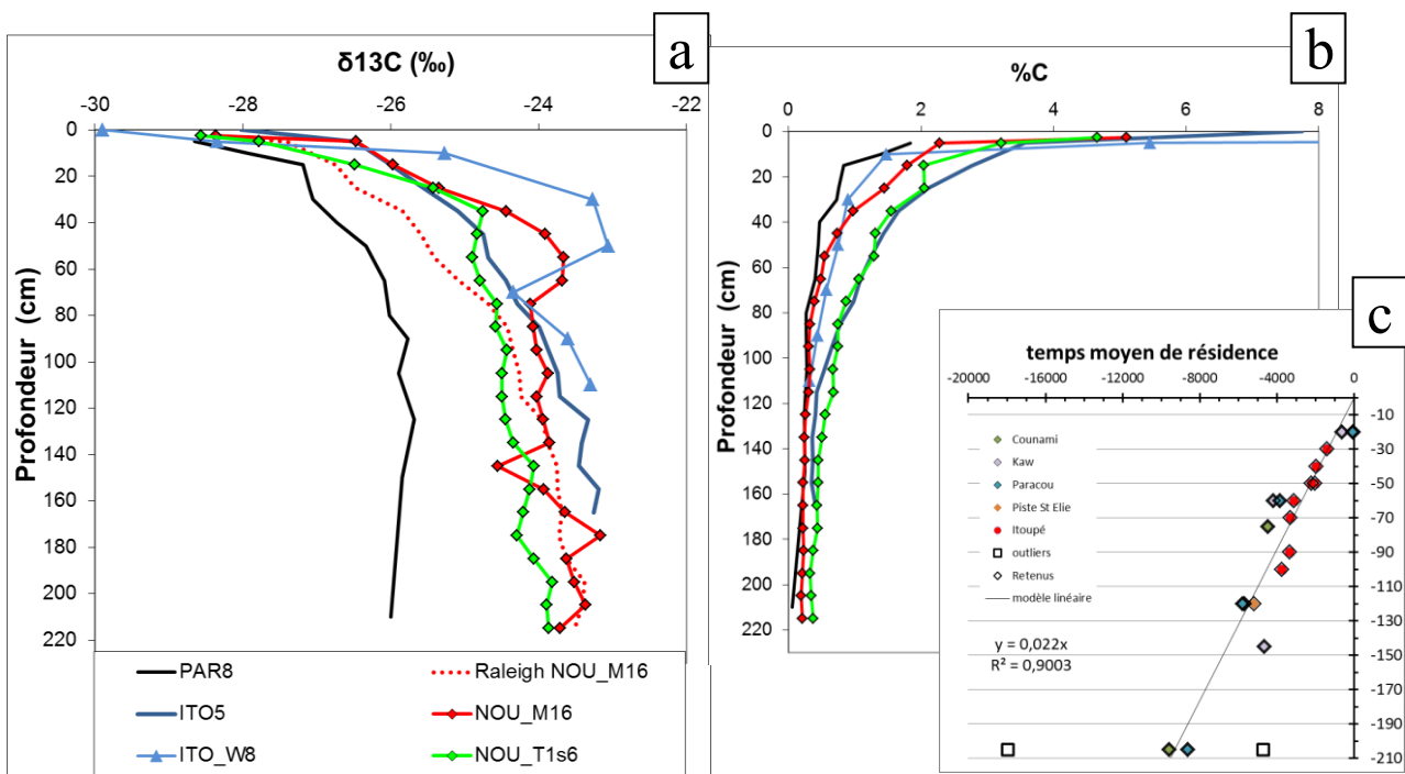
Fig. 20. a) Exemple de profils \delta^{13}\text{C} de la matière organique des sols ; PAR8 et ITO5 montrent les variations extrêmes attribuables aux conditions pédologiques (Wynn et al. 2005) ; ITO_W8, NOU_M16 et T1s6 montrent au contraire à faible profondeur un pic plus ou moins prononcé qui s'écarte du modèle théorique de Raleigh, représenté pour NOU_M16 ; b) Les concentrations en carbone diminuent fortement et régulièrement avec la profondeur ; c) Datation ^{14}\text{C} des temps moyens de résidence de la MOS en fonction de la profondeur (cm) ; en rouge, datation des bornes des pics de trois profils à ITO_W.
