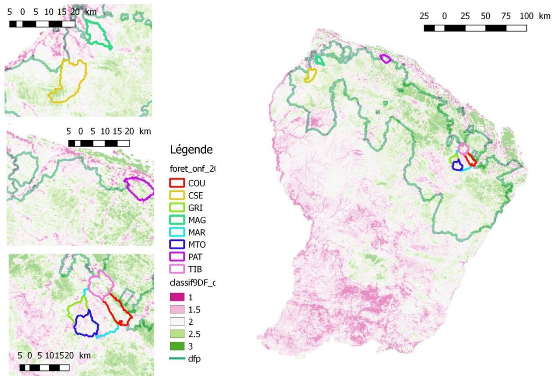
Fig. 26. Massifs forestiers du DFP (Domaine Forestier Permanent) pour lesquels au moins 15 parcelles ont été exploitées au cours de la période 1995-2005 ; classif9DF : scores de la classification Landsat « dynamique ».
