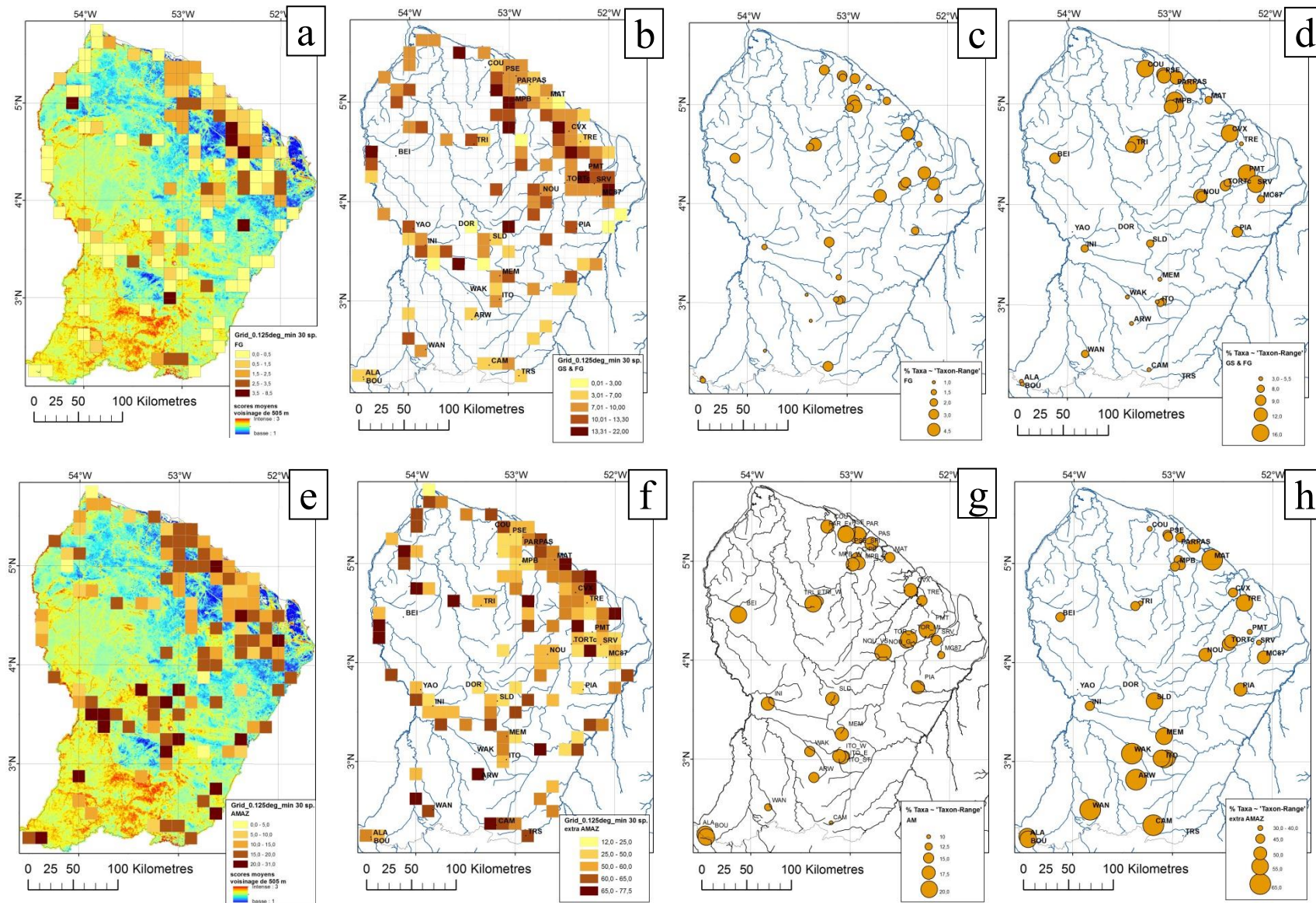
Fig. 25. Contribution des espèces arborescentes aux flores locales, d'après les collections d'herbiers (a, b, e, f) et aux communautés, d'après les inventaires Guyadiv (c, d, g, h), en fonction de leur aire de distribution ; FG : Guyane française (a, c) ; GS : Guyanes (b, d) ; AMAZ : Amazonie (e, g) ; extraAMAZ : Amazonie et hors d'Amazonie (f, h).
