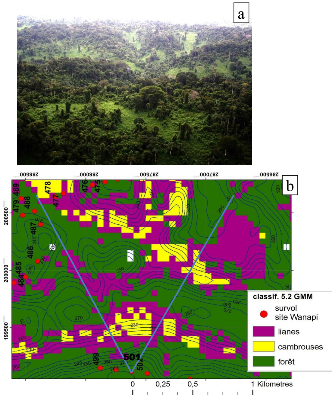
Fig. 9. a) Paysage à canopée ouverte, cambrousques et lianes au site Wanapi (prise de vue n° 501 D. Sabatier) ; on note au premier plan les arbres isolés portant des manchons de lianes ; b) Extrait de la classification supervisée thématique de l'image Landsat au site Wanapi ; les lignes indiquent approximativement le champ de visée du cliché 501.
