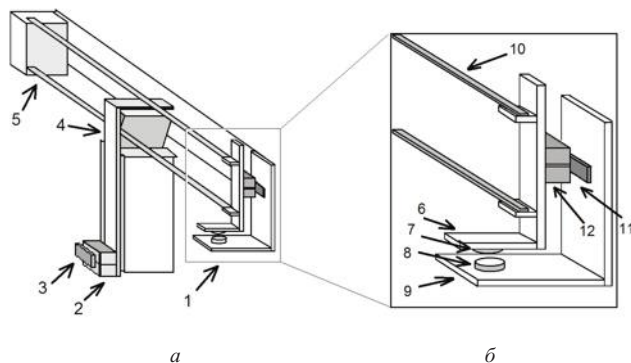
а – датчик изменения массы высечки листа: 1 – плечо весов с датчиком толщины листа, 2 – пара магнитов, 3 – датчик Холла, 4 – балансир, 5 – плечо весов с закреплением пружин; б – датчик изменения толщины высечки листа: 6 – верхняя опорная площадка, 7 – верхняя контактная поверхность, 8 – нижняя (неподвижная) контактная поверхность, 9 – нижняя опорная площадка, 10 – пружина, 11 – датчик Холла, 12 – пара магнитов
