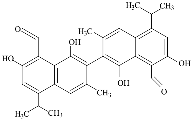
Gossypiol
