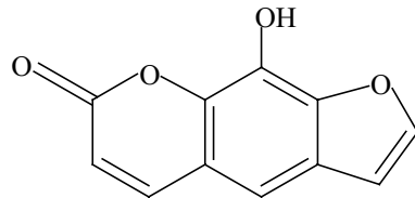
Xanthotoxol
