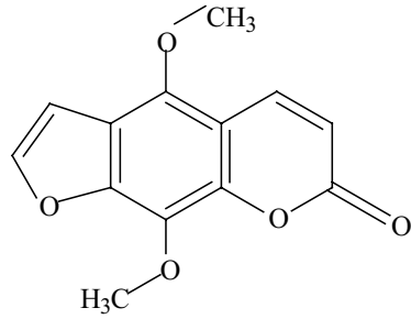
Isopimpinellin
