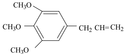
Elemicin
