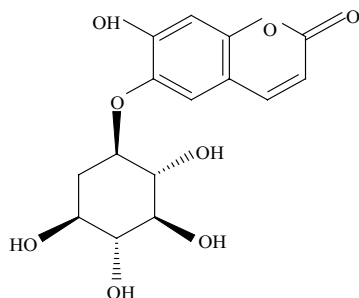
Fig. 15.4 Esculin.
