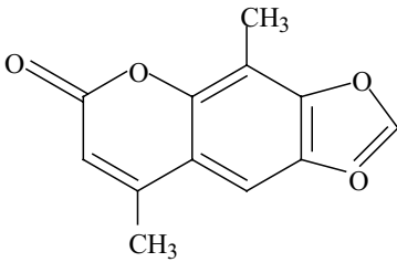
Trioxsalen
