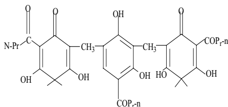
Filixic acid
