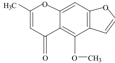
Visnagin
