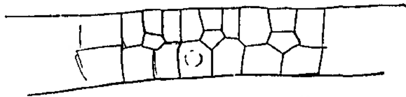
Fig. 3. Polysiphonia (Placophora) Bideri, optischer Querschnitt eines Flachsprosses.
