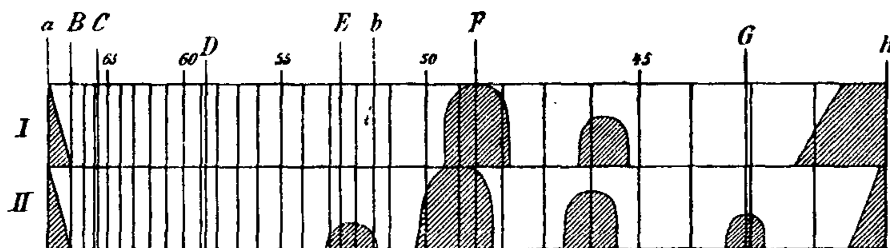
Absorptionsspectren gelber Fettfarbstoffe. I. Spectrum eines gewöhnlichen gelben Lipochroms mit seinen zwei Bändern. II. Spectrum des Lipochroms der Lycogala -Arten mit 4 Bändern (verdünnte Petrolätherlösung des gereinigten Farbstoffes; 60 mm Schichtenhöhe; Sonnenlicht).
