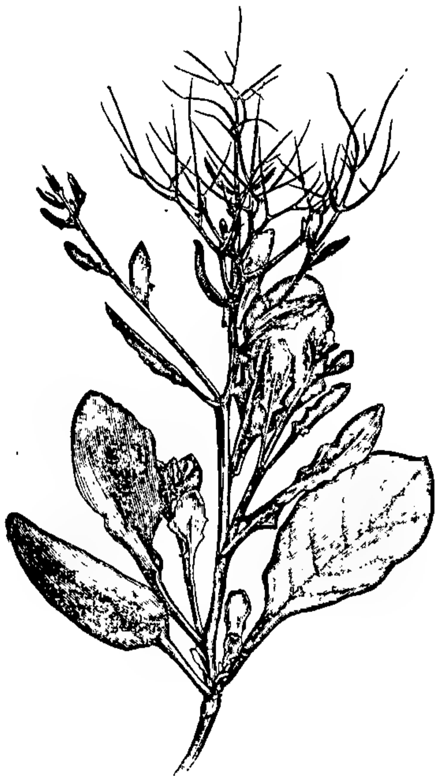
Fig. 5. Zylla myagroïdes Keimpflanze, unten mit grossen Laubblättern, oben mit schuppenförmigen (in der Figur nicht sichtbaren) Blättern. Etwa d. Hälfte d. nat. Gr.
