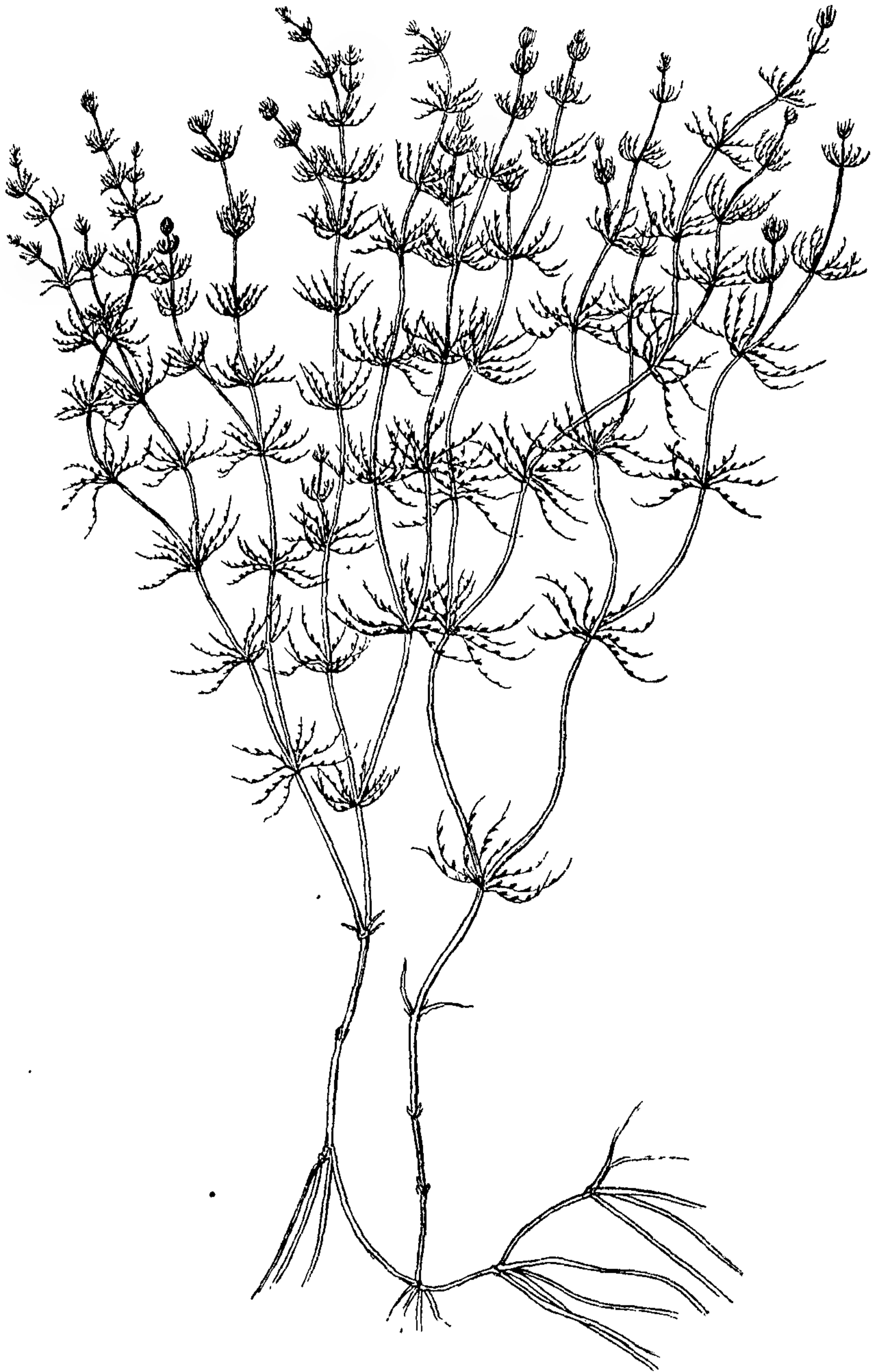
Fig. 1. Chara foetida A. Br. Habitusbild. Originalzeichnung.
