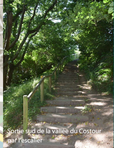
Vallée du Costour - Vannes du bassin
