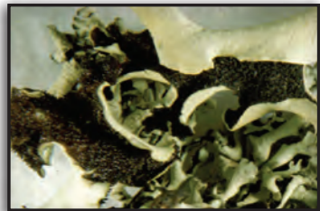
X. neochlorochroa
