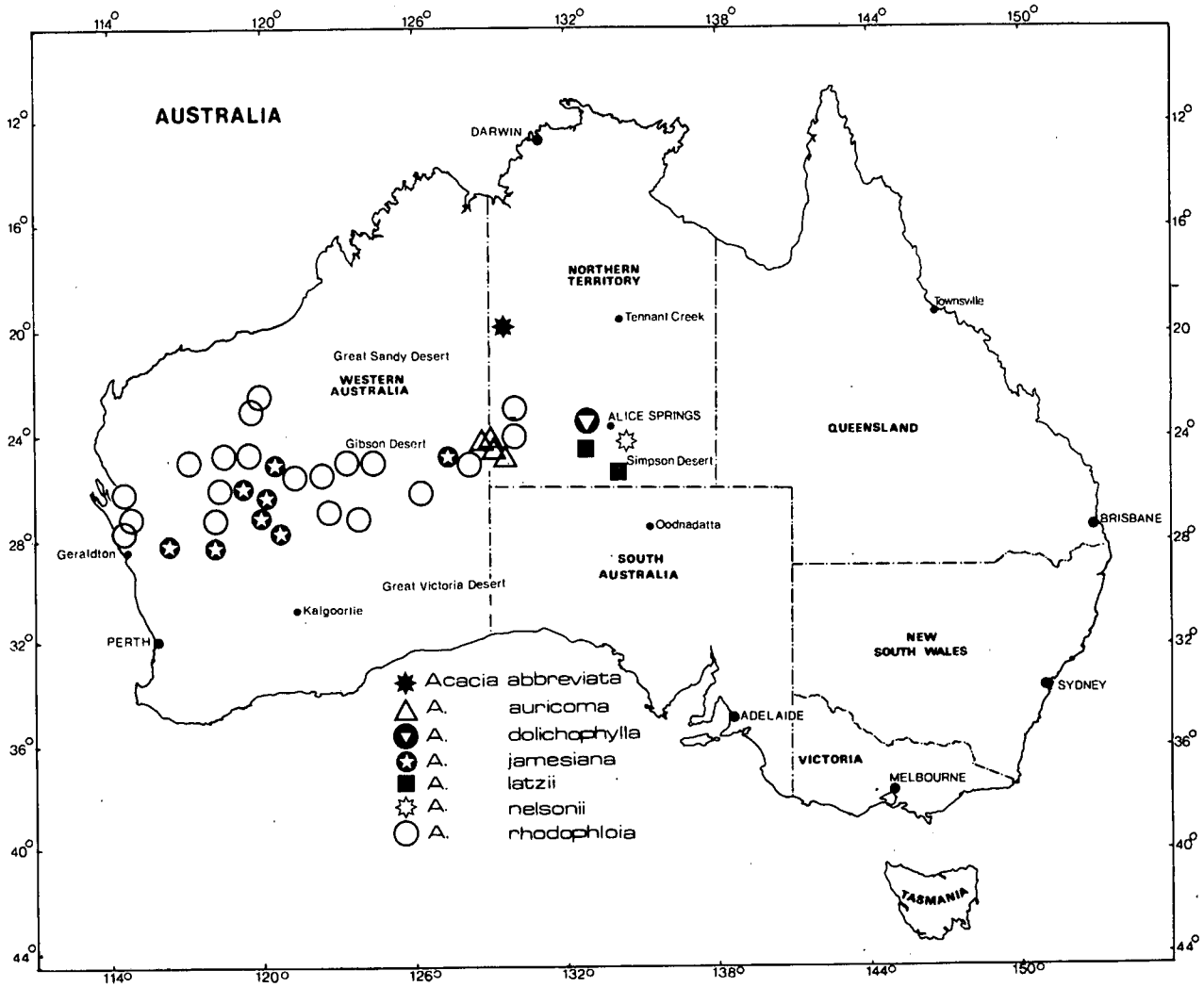
Fig. 8. Distribution map of Acacia abbreviata , A. auricoma , A. dolichophylla , A. jamesiana , A. latzii , A. nelsonii and A. rhodophloia .
