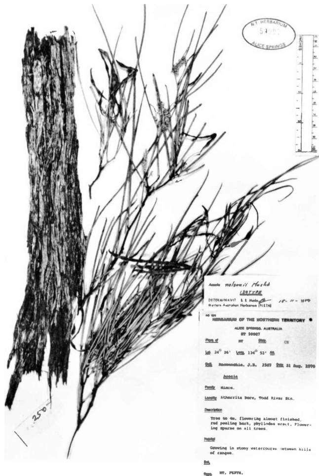
Fig. 6. Acacia nelsonii sp. nov. (J.R. Maconochie 2507, isotype—NT).
