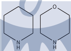
Аміни
