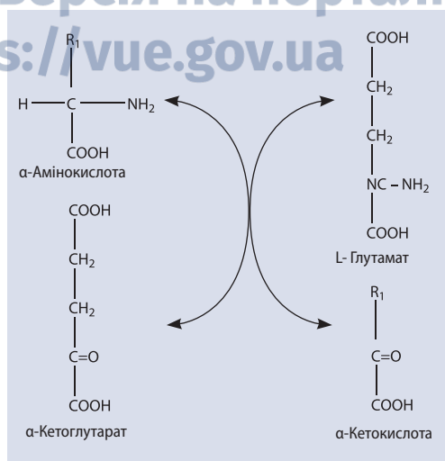
Аміотрансферази. Загальна схема реакції трансамінування
