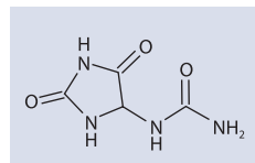
Алантаїн. Рис. 1. Структурна формула
