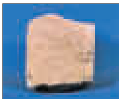
Алевроліт
