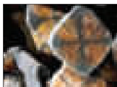
Андалузит
