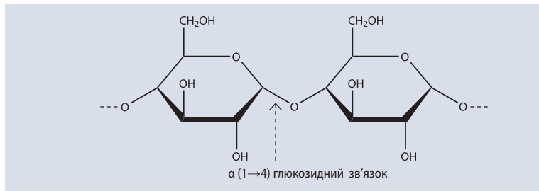
Амілоза
