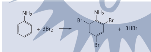
Анілін. Реакція якісного і кількісного визначення аніліну
