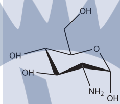
Аміноцукри
