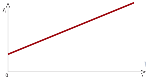
Аналіз часових рядів. Гіпотетичний часовий ряд, що містить зростаючу тенденцію
