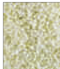
Аміачна селітра
