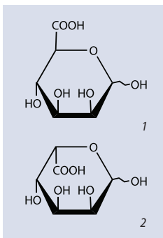
Альгінові кислоти. Структурні формули D-мануранової (1) та L-гулуранової (2) кислот
