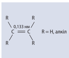
Алкєни
