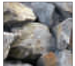
Андезит
