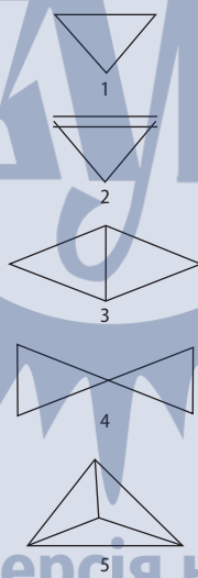
Аліциклічні сполуки
