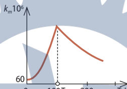
Антиферомагнетизм. Повна залежність магнітної сприйнятливості \chi_m від температури для MnO. Температура Нееля тут T_n = 120 К
