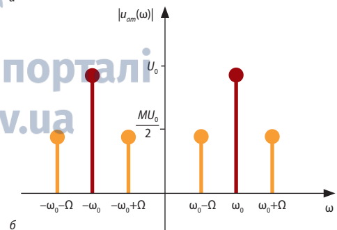
Амплітудна модуляція. Часова залежність амплітуди (а) і амплітудний спектр (б) АМ сигналу з однотонольною амплітудною модуляцією. U_0 , \omega_0 — амплітуда й частота сигналу-носія, \Omega — частота модулюючого сигналу, U(t) — об'єднана, U_{max} , U_{min} — максимальне й мінімальне значення амплітуди АМ сигналу
