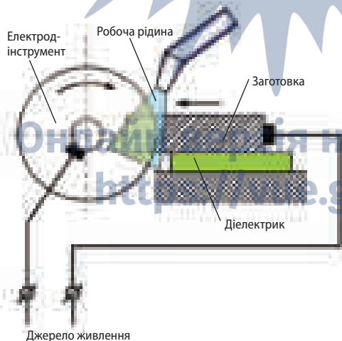
Анодно-механічна обробка. Схема анодно-механічної обробки
