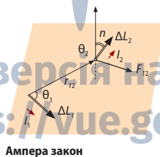
Ампера закон
