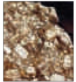
Андезит
