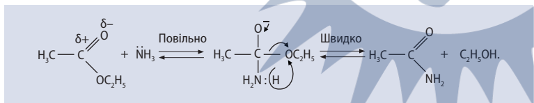
Амоніліз. Механізм амонілізу етилetanoату
