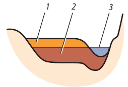
Алювій.
