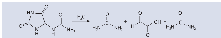
Алантаїн. Рис. 5. Гідроліз
