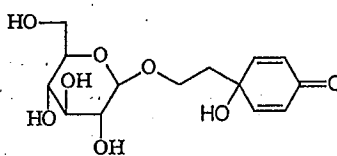
2 comoside
