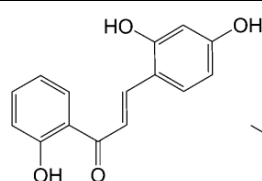
Isoliquirtigenin (47)
