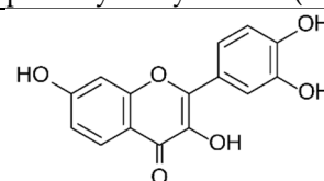
Fisetin (42)
