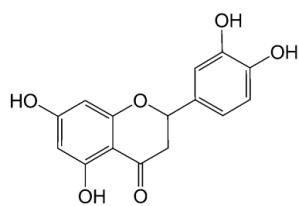
Eriodictyol (37)
