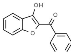
Auronol (32)
