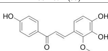
Licochalcones (56)
