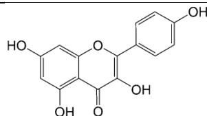
Kaempferol (23)
