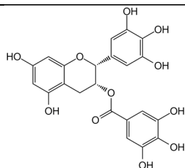
EGCG (20)
