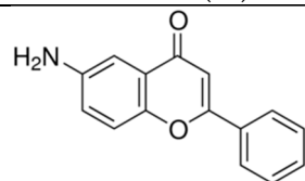
6-aminoflavone (28)
