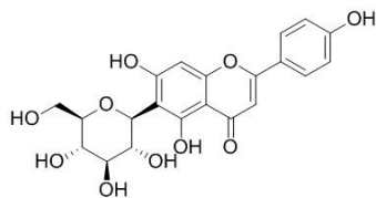
Isovitexin (19)
