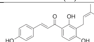
Nobiletin (51)
