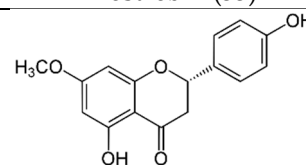
Pinostrobin (33)
