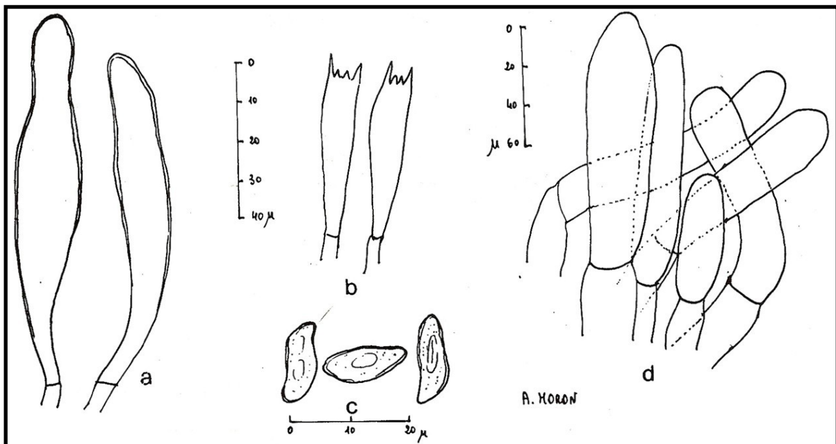
Boletinus asiaticus : a = cistidi; b = basidi; c = spore; d = cuticola
