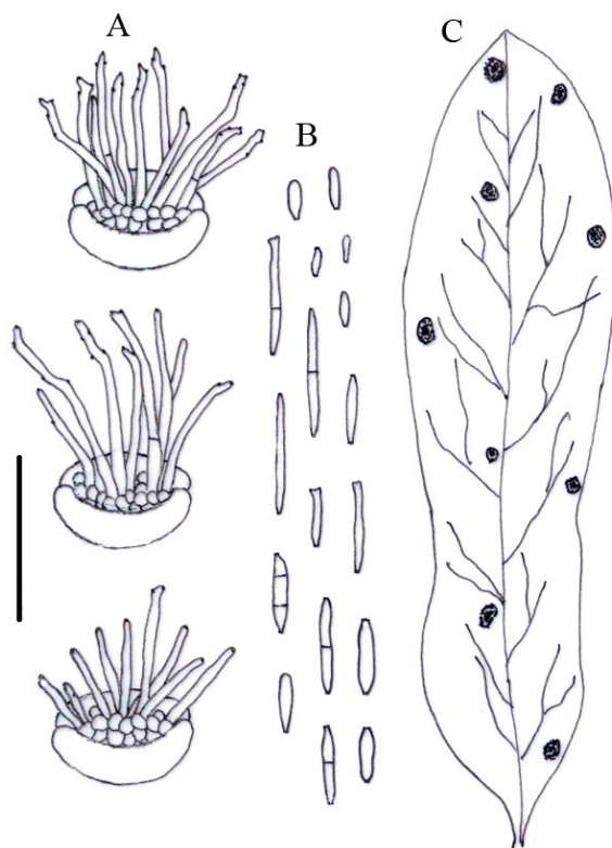
شکل ۳- Ramularia pratensis var. pratensis روی Rumex crispus : A. کنیدیوفورها، B. کنیدیوم‌ها (مقیاس = ۵۰ میکرومتر)، C. علائم روی برگ.
