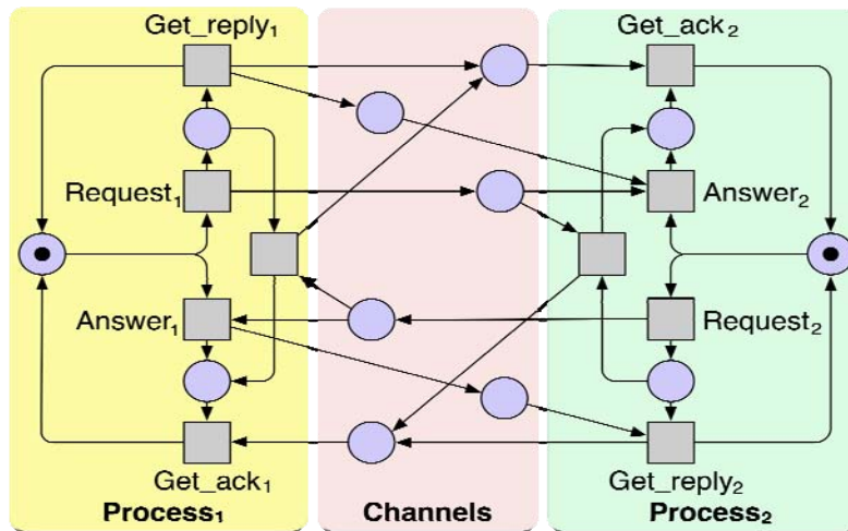
Petrietzmodell eines einfachen Kommunikationprotokolls
