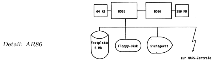
Teilsystem C: MARS-Verbund
