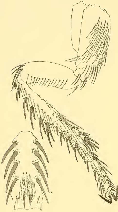
Fig. 10. Außenseite eines fünften Tarsalgliedes des dritten Beines.
