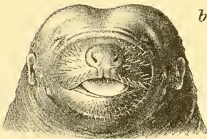
Fig. 1. Erinaceus europaeus L.; Embryo, gesammelt von Professor Hochstetter. \times 1\frac{1}{2} .
