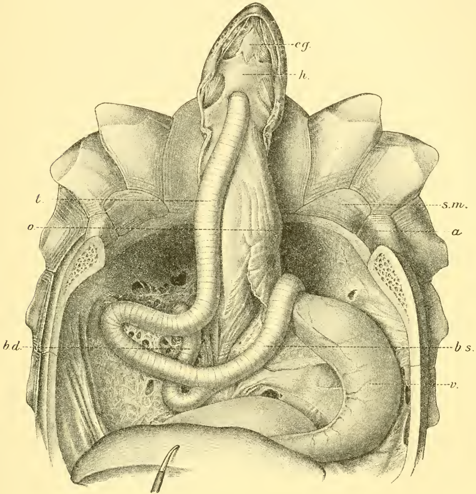
Cinixys erosa Schw., ♀, \frac{1}{5} nat. Gr.
