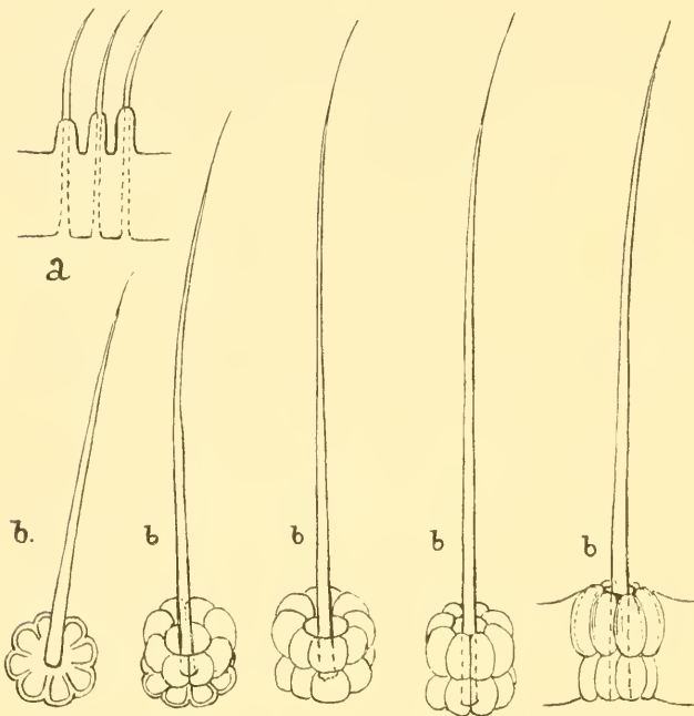
Fig. 5. Sinnesorgane des achten Tergites.
