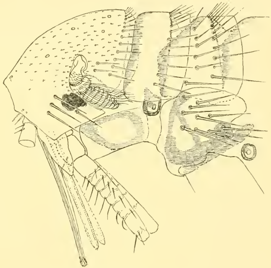
Fig. 4. Kopf der Vermipsylla hyaenae Kol. ♀.
