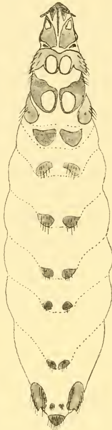
Fig. 3. Bauchansicht desselben Individuums.
