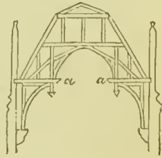
a. Hammer-beam.
