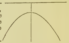
Directrix.
