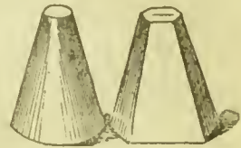
Frustum.
