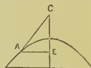
Subtangent
