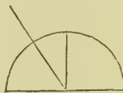
Cosecant.
