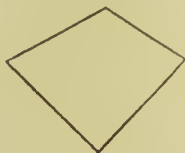
Trapezium.
