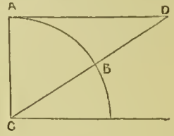
Secant.
