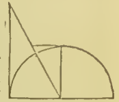
Cotangent.
