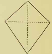
Deltoid.
