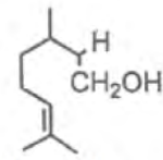
Citronelol
