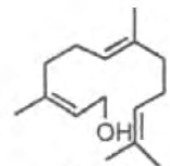
Farnesol
