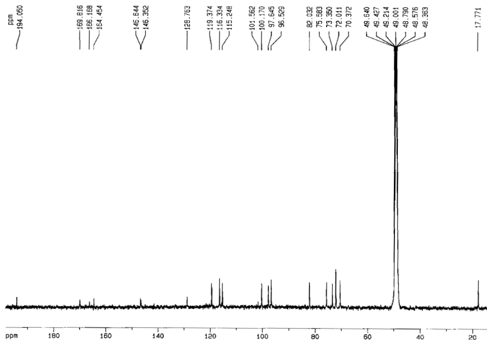
Figura 9. Espectro de RMN ^{13}\text{C} da neoisoastilbina ( \text{CD}_4\text{O} , 50 MHz).
