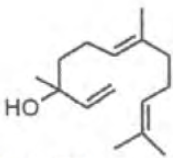
Nerolidol
