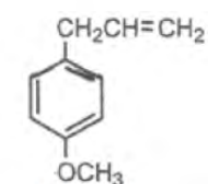
Estragol
