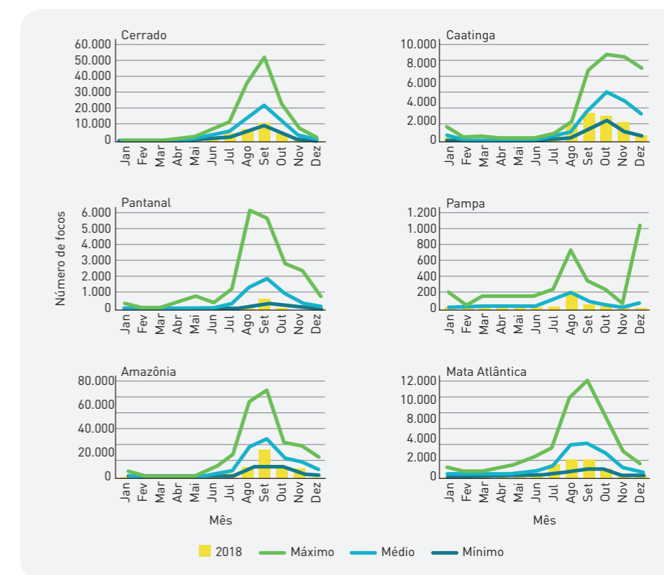
Figura 3.24. Focos ativos de queimadas observados nos biomas brasileiros entre os anos de 1998 e 2018. Dados obtidos do Instituto Nacional de Pesquisas Espaciais/INPE (2018).
