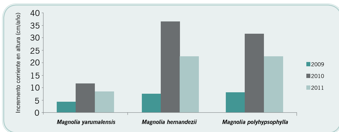
Figura 4. Representación gráfica del incremento corriente anual en los 3 primeros años para 3 especies de Magnolia establecidas en campo abierto
