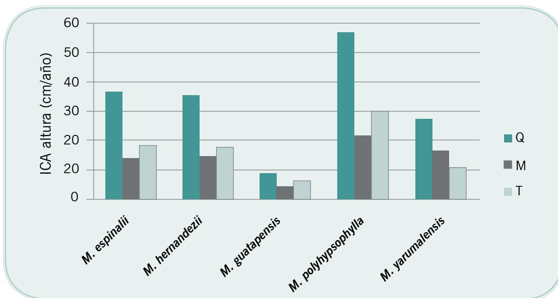
Figura 1. Representación gráfica del ICA en altura, por especie y subsidio
