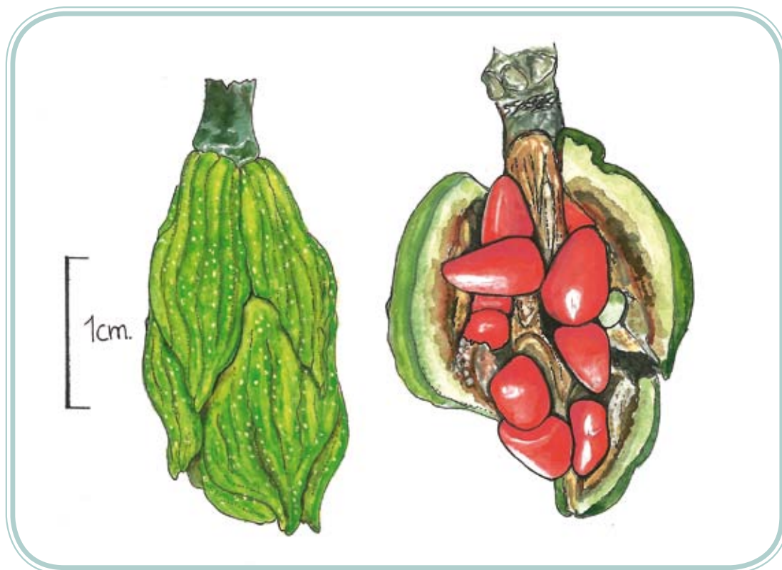
Figura 3. Detalle del fruto de almanegra ( Magnolia guatapensis )
