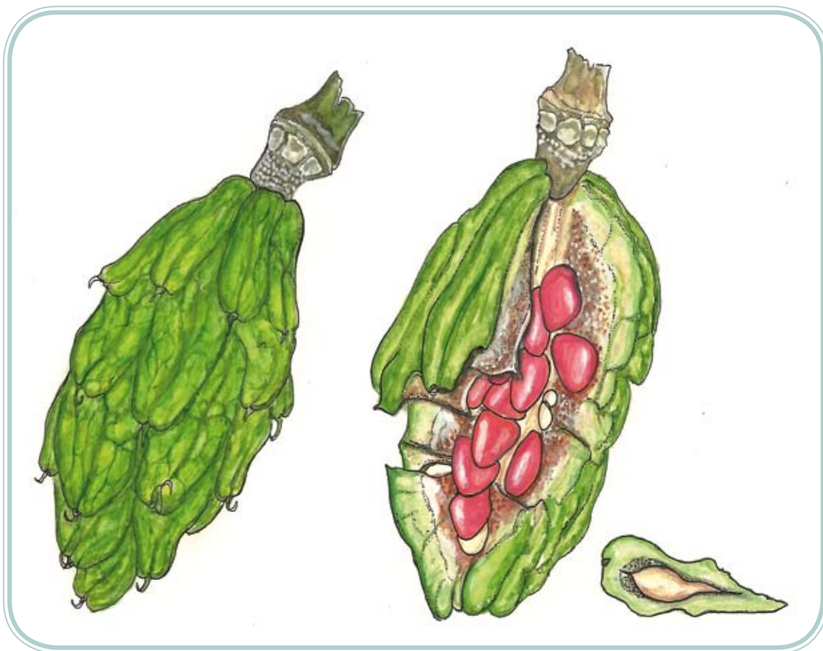
Figura 9. Detalle del fruto de gallinazo morado ( Magnolia yarumalensis )
