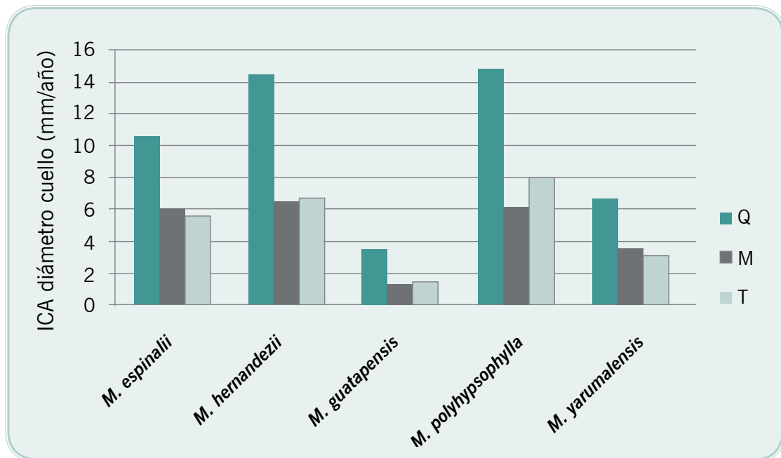
Figura 2. Representación gráfica del ICA en diámetro del cuello radicular, por especie y subsidio
