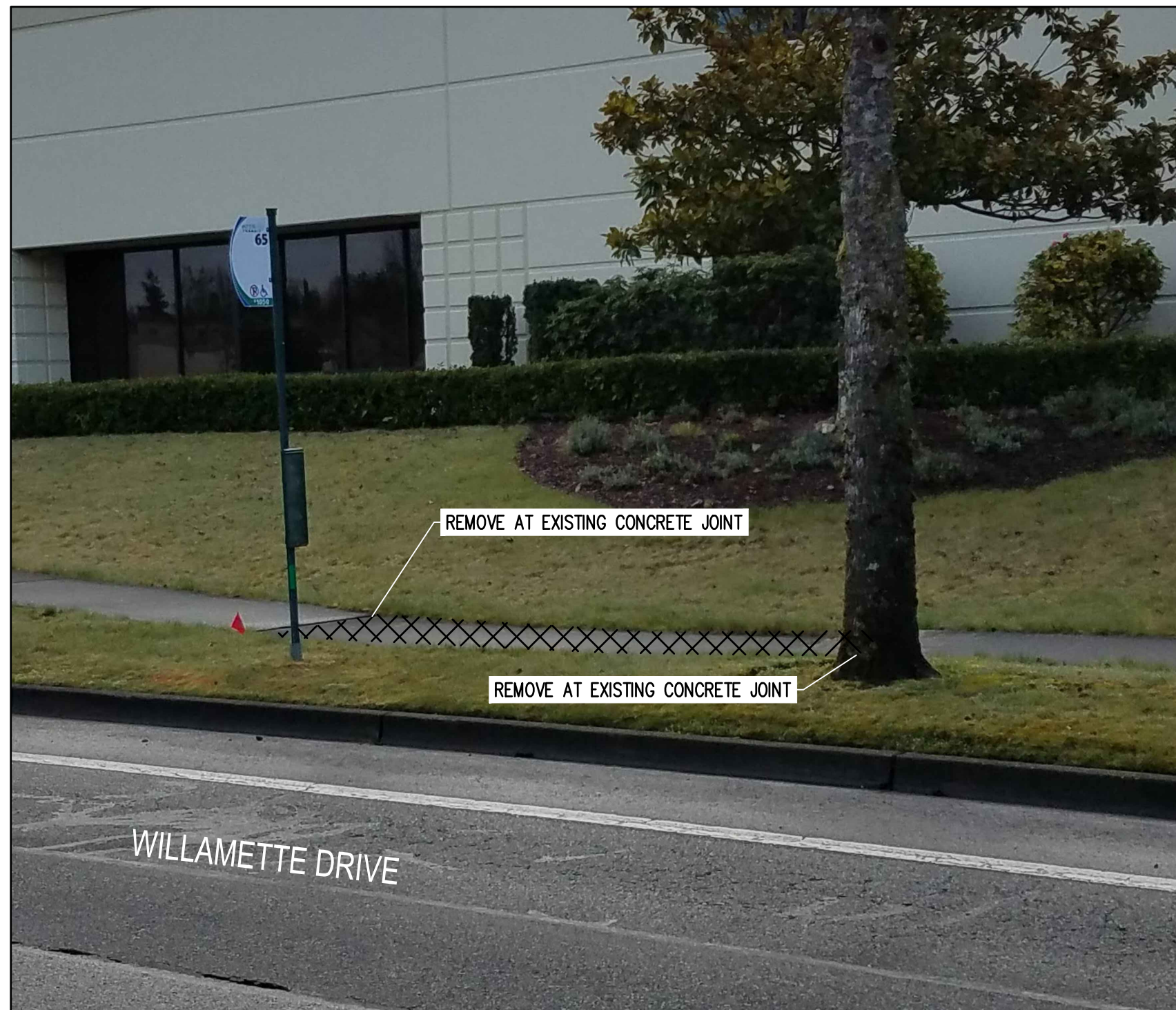
EXISTING CONDITIONS N.T.S.
