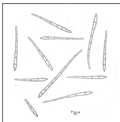
Conidiophores et conidies de P. fijiensis
