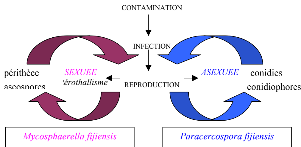
Figure 1 : cycle infectieux de M. fijiensis (d'après Mourichon et al. , 1997)
