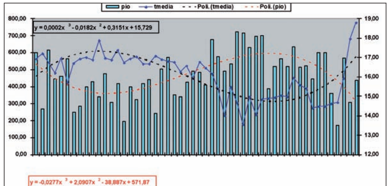
Figura 7: Diagramma termo-pluviometrico con le variazioni pluriennali delle temperature medie annue messe a confronto con le precipitazioni totali annue alla stazione di Pianosa (1951-2002).
