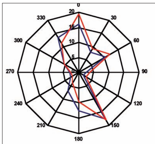
Figura 8: Distribuzione delle frequenze medie percentuali in relazione alle direzioni principali della Rosa dei Venti. Dati 2002-2003, CNR-IBIMET.
