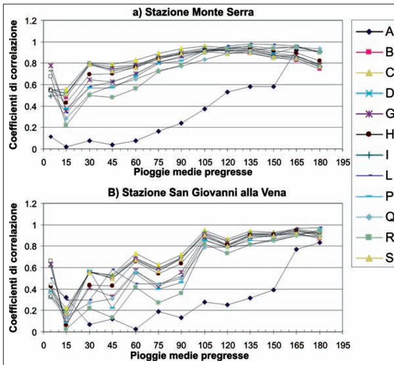
Figura 8: Diagrammi dei coefficienti di correlazione freatimetria contro l'intervallo temporale di precipitazione media pregressa per le stazioni di a) Monte Serra e b) San Giovanni alla Vena.
