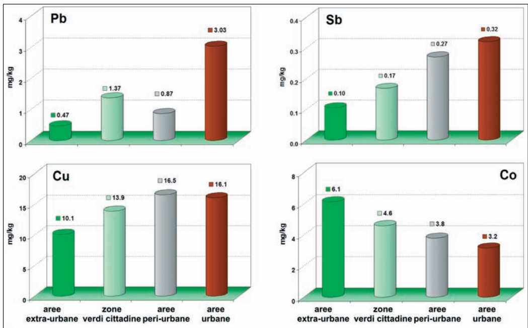
Figura 5: Concentrazioni medie di Pb, Sb, Cu e Co nei lombrichi di Siena.
