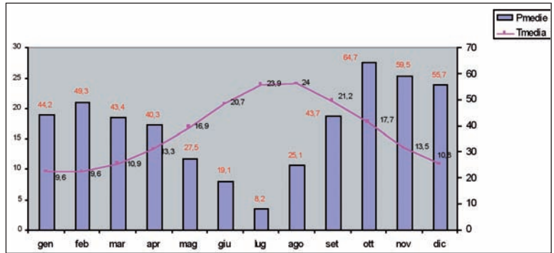
Figura 6: Diagramma termo-pluviometrico delle medie mensili calcolate nel periodo 1951-2002 (Pianosa).
