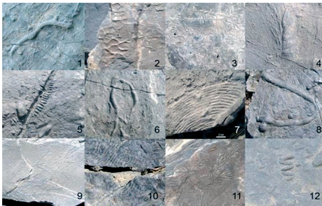
Figura 3: Esempi di icnofossili dal Cretaceo superiore del Rio Ardenza (Livorno).
