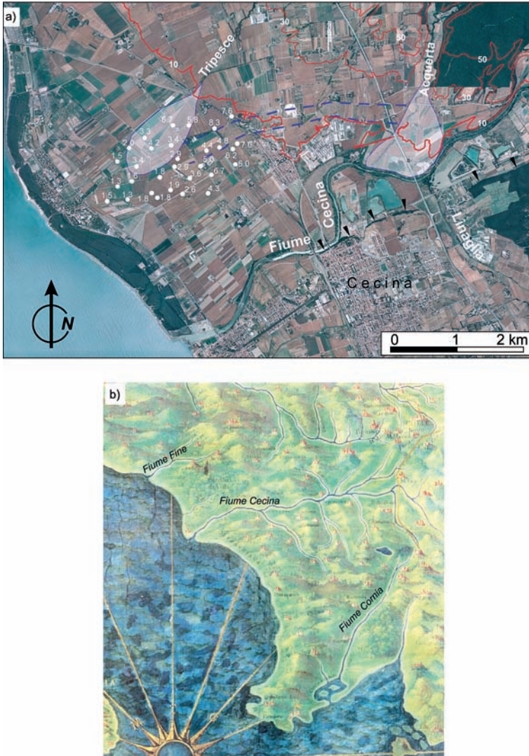
Figura 3: (a) Foto aeree del corso terminale del Fiume Cecina. I triangoli neri indicano la scarpata morfologica. La linea tratteggiata indica l'antico corso del Cecina. I coni alluvionali dell'Acquerta e del Tripesce. (b) Parte della Carta Etruria di Egnazio Danti che illustra la Toscana costiera fra i fiumi Fine e Cornia, sulla quale è evidente delta del Fiume Cecina [10].
