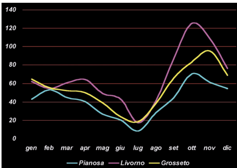
Figura 4: Diagrammi delle precipitazioni medie mensili nel periodo 1960-2000 elaborate dai dati delle stazioni di Pianosa, Livorno e Grosseto.
