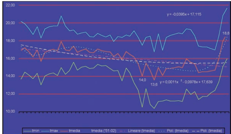
Figura 3: Diagramma delle temperature medie annue registrate a Pianosa nel periodo 1951-2002. Sono indicate la retta e le curve di tendenza (II e VI ordine), con le relative equazioni, e la media normale.
