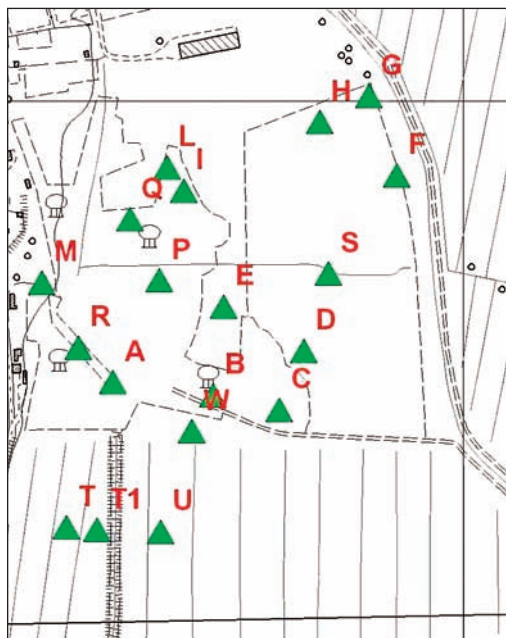
Figura 3: Ubicazione dei sondaggi stratigrafici e piezometri.
