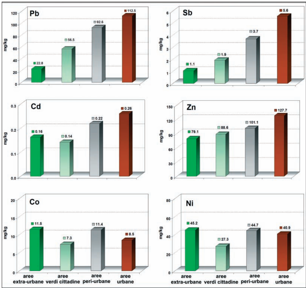
Figura 2: Contenuti medi di Pb, Sb, Cd, Zn, Co e Ni nei suoli dell'area di studio.
