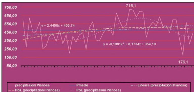
Figura 5: Precipitazioni annue a Pianosa nel periodo 1951-2002. Sono indicate la retta e le curve di tendenza (II e VI ordine), con le relative equazioni, e la media normale.
