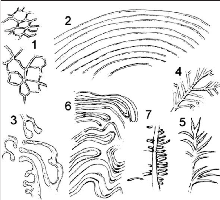
Figura 4: Schemi di icnofossili dal Rio Ardenza. 1, agricchnia ( Paleodictyon isp.); 2, agricchnia ( Spiroraphe isp.); 3, agricchnia (cfr. Graphoglyptid isp.); 4-5, fodinichnia ; 6, fodinichnia ; 7, probabile repichnia (cfr. Gyrolithes isp. attraversato da frattura).
