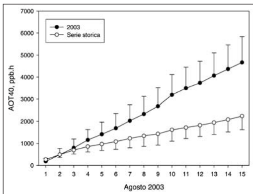
Figura 1: valori giornalieri di AOT40, osservati in nove stazioni di monitoraggio toscane nel periodo 1-15 agosto 2003, confrontati con la rispettiva serie storica (1999-2002 + 2004). Le barre verticali indicano le deviazioni standard delle medie [4].
