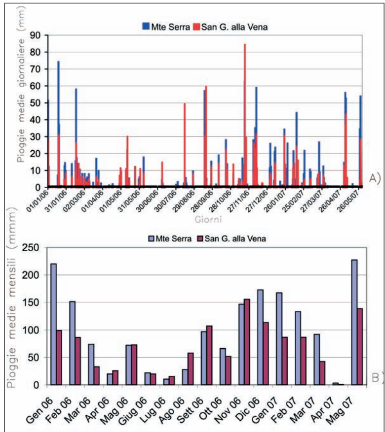
Figura 7: Istogramma piogge medie A) giornaliere e B) mensili per le stazioni di Monte Serra e San Giovanni alla Vena.
