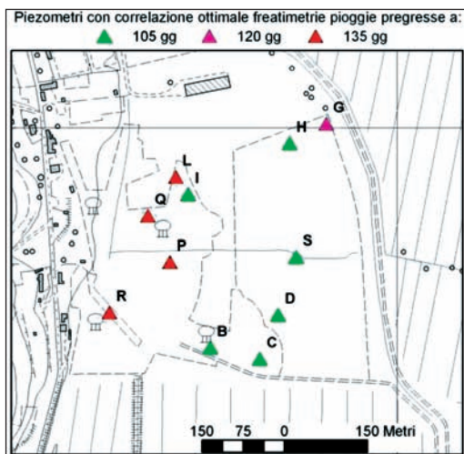
Figura 9: Raggruppamento areale di piezometri a comportamento simile. In rosso freatimetrie a correlazione ottimale a 105 gg, in verde freatimetrie a correlazione ottimale a 135 gg in blu piezometro G a correlazione ottimale a 120 gg.
