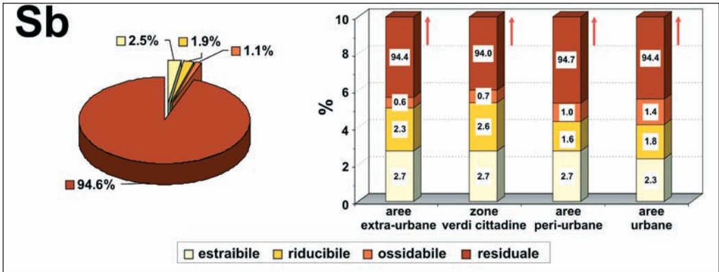
Figura 4: Frazionamento dell'antimonio nei suoli dell'area di studio.
