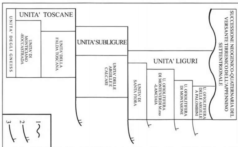
Schema dei rapporti stratigrafico-strutturali delle unità presenti nella toscana meridionale: i. contatto stratigrafico erosivo. ii. sovrascorrimento primario. iii. sovrascorrimento secondario.
