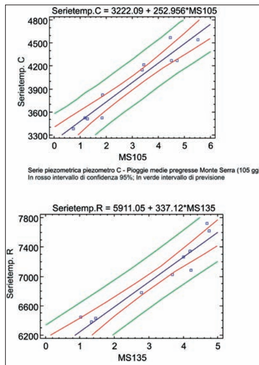
Figura 10: Diagrammi di regressione altezze freatimetriche - precipitazioni medie pregresse (105 gg per piezometro C e 135 gg per piezometro P).
