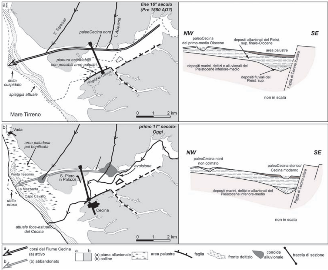
Figura 5: Evoluzione del drenaggio del Fiume Cecina alla fine del 16° secolo e all'inizio del 17° secolo, e relative sezioni geologiche schematiche, non in scala.
