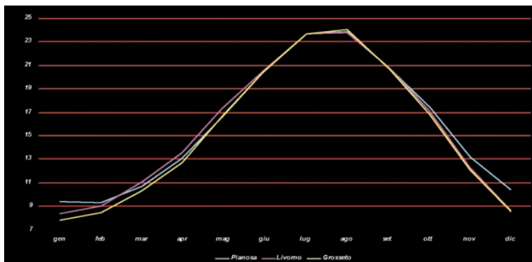
Figura 1: Diagrammi delle temperature medie mensili nel periodo 1960-2000 elaborate dai dati delle stazioni di Pianosa, Livorno e Grosseto.
