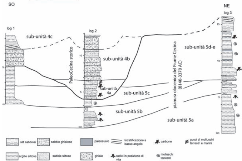
Figura 4: (a) Localizzazione e (b) correlazione di tre sezioni stratigrafiche misurate in una cava attiva presso Cecina, sulle unità 4 e 5.
