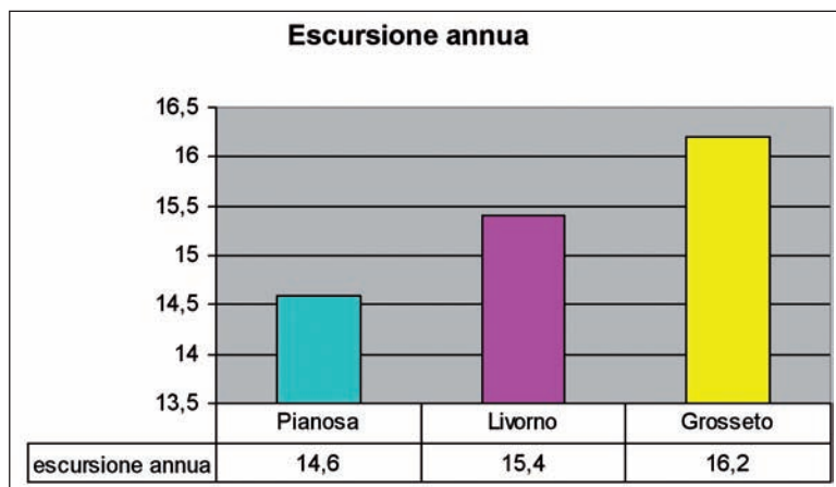
Figura 2: L'escursione annua alle stazioni marittime di Pianosa, Livorno e Grosseto (1960-2000).
