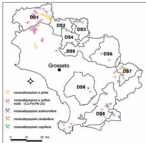
Figura 2: Ubicazione dei principali siti mineralari presenti nell'area di studio.
