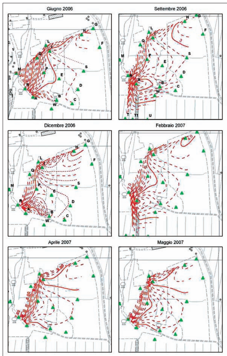
Figura 6: Carte delle freatimetrie.
