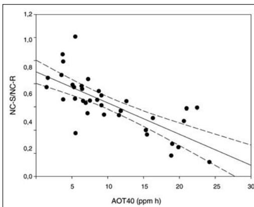
Figura 5: Associazione tra il rapporto della biomassa epigea di NC-S e quella di NC-R di trifoglio bianco e l'AOT40 nel periodo 1997-2006 a Pisa; le linee tratteggiate indicano gli intervalli di confidenza ( p < 0,05 ) ( y = 9,03e^{-1} - 2,69e^{-5} x , R^2 = 0,55 ).
