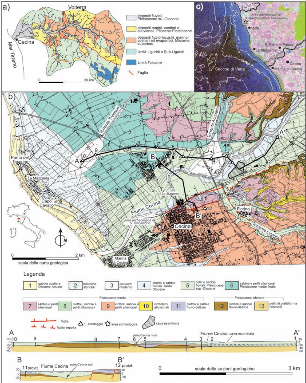
Figura 1: (a) Carta geologica semplificata del bacino idrografico del Fiume Cecina. (b) Carta geologica dell'area di studio (modificata dai rilevamenti degli autori per il Servizio Geologico della Regione Toscana). (c) Batimetria delle Secche di Vada [3].
