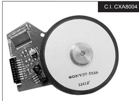
MV 497 MOTOR DE CAPSTAN
