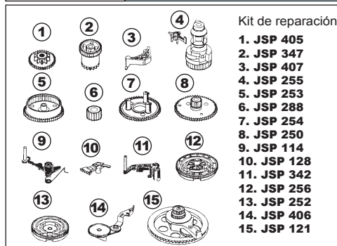
JSP 702 KIT DE REPARACION
