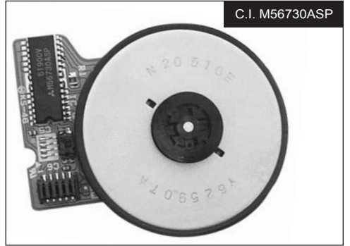
MV 326 MOTOR DE REBOBINADO
