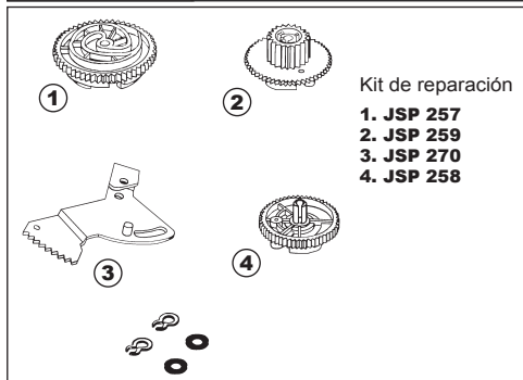
JSP 701 KIT DE REPARACION
