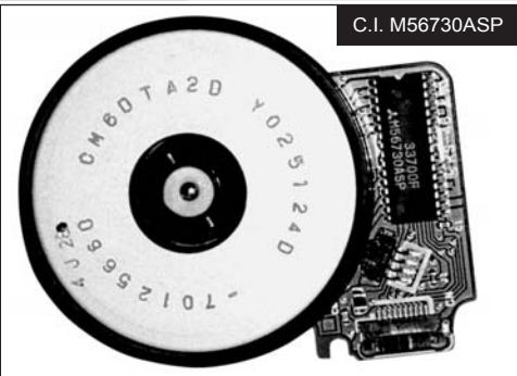
MV 458 MOTOR DE CAPSTAN
