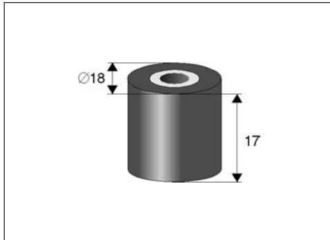
JSP 079 ENGRANAJE
