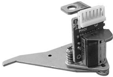
CV 333 CABEZA DE AUDIO. CTL
