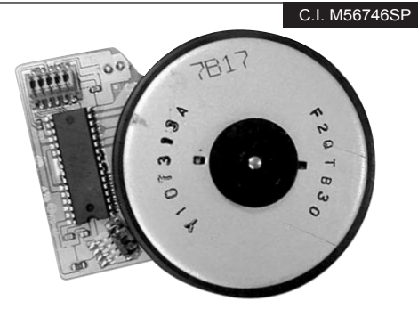
MV 607 MOTOR DE CARGA
