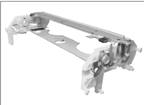
JSP 1264 FRENO
