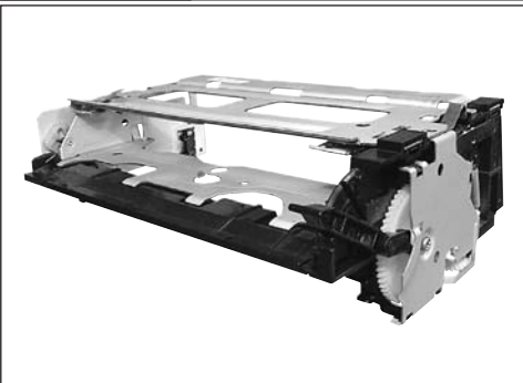
JSP 1382 ENGRANAJE
