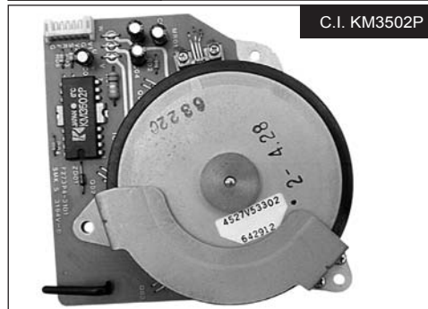
MV 361 MOTOR DE CAPSTAN
