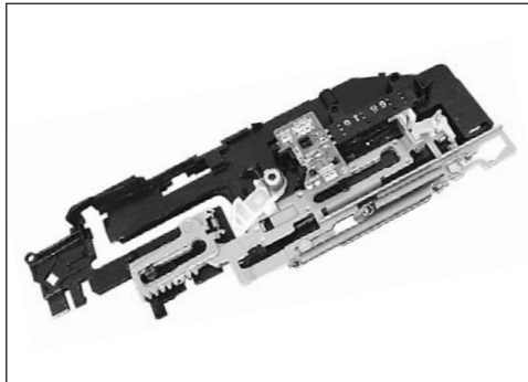
JSP 398 ENGRANAJE
