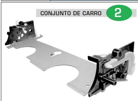
JSP 1280 CONJUNTO DE CARRO 2
