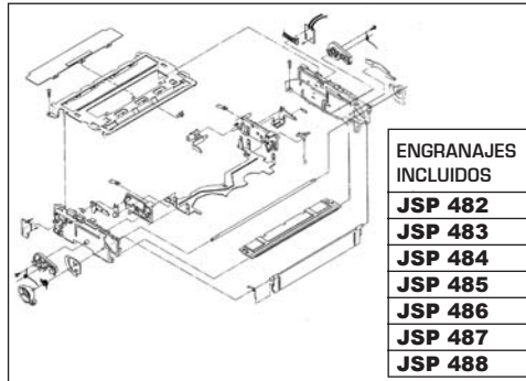
MV 418 MOTOR DE CARGA
