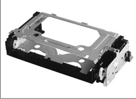
JSP 997 FRENO
