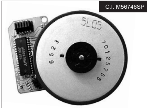
MV 533 MOTOR DE CAPSTAN
