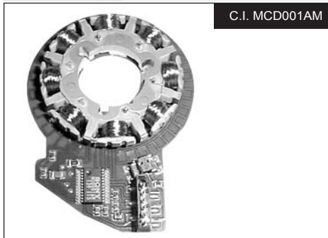
MV 495 MOTOR DE CABEZAS
