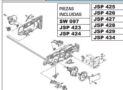
JSP 551 CARRO
