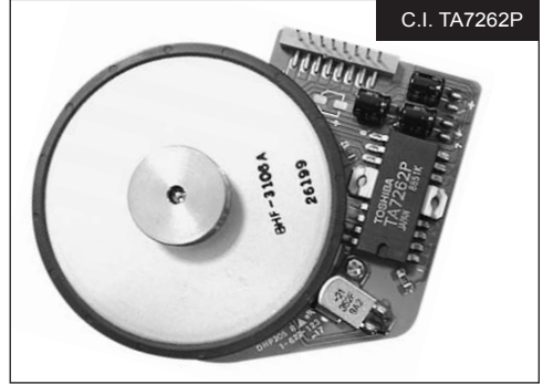
MV 381 MOTOR DE CAPSTAN
