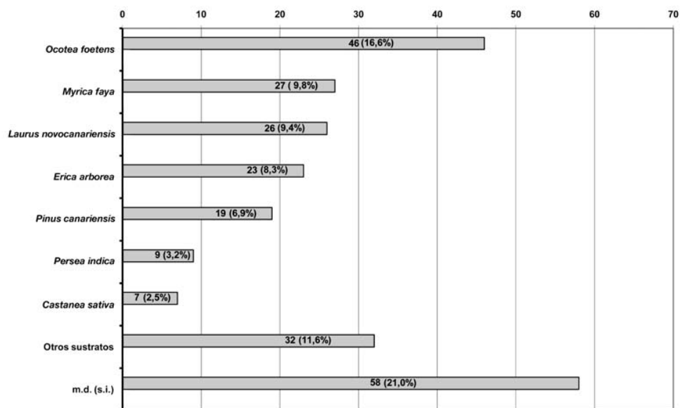
Fig. 7. Número de especies y porcentajes recolectadas en las diferentes especies de plantas vasculares sustratos
