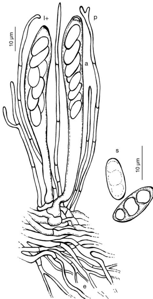
Fig. 3. Discinella aff. boudieri : a, ascas; p, parafisos; s, esporas; e, células del excípulo medular (dibujos de L. Quijada).
