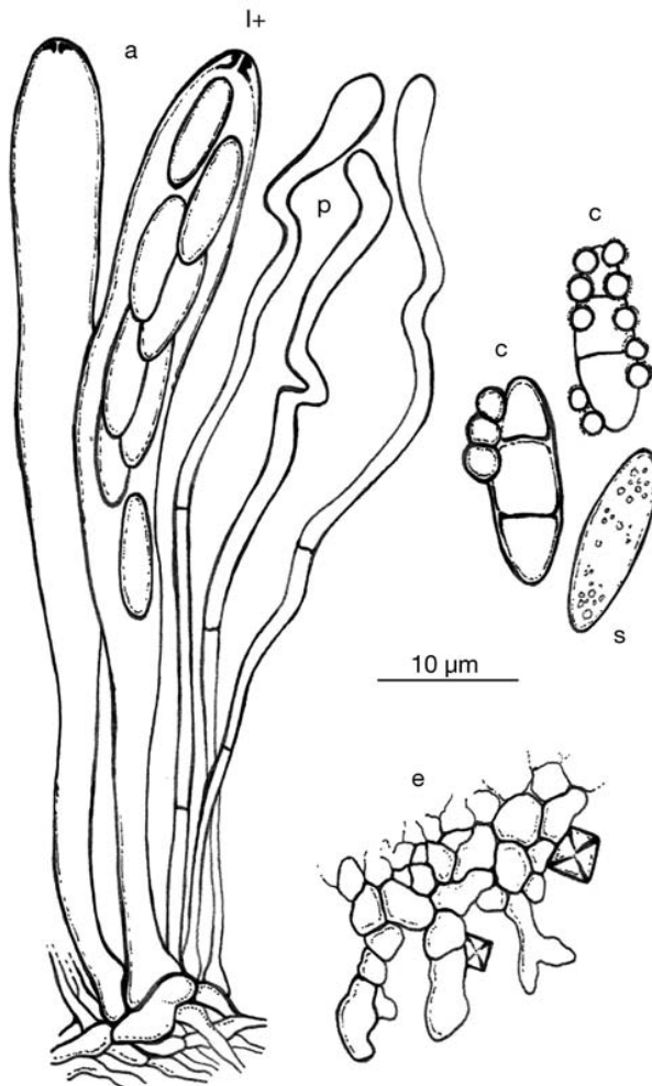
Fig. 2. Ascocoryne aff. cylichnium : a , ascas; p , parafisos; s , esporas; c , conidios; e , células del excípu-lo ectal (dibujos de L. Quijada).
