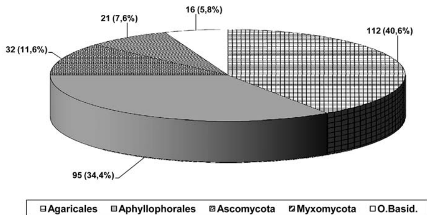
Fig. 5. Número de especies y porcentajes respectivos, pertenecientes a los diferentes grupos fúngicos estudiados.
