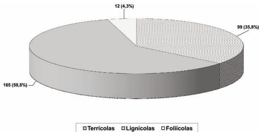
Fig. 6. Número de especies y porcentajes, de los diferentes grupos fúngicos, atendiendo a las distintas categorías ecológicas respecto a los sustratos.
