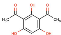
2,4 diacetyl phloroglucinol
