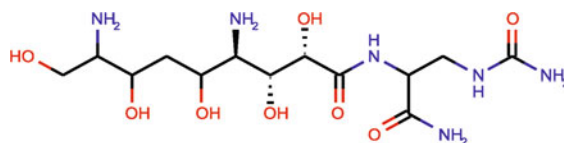
zwittermycin A
