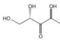
4,5 dihydroxy 2,3 pentadione
